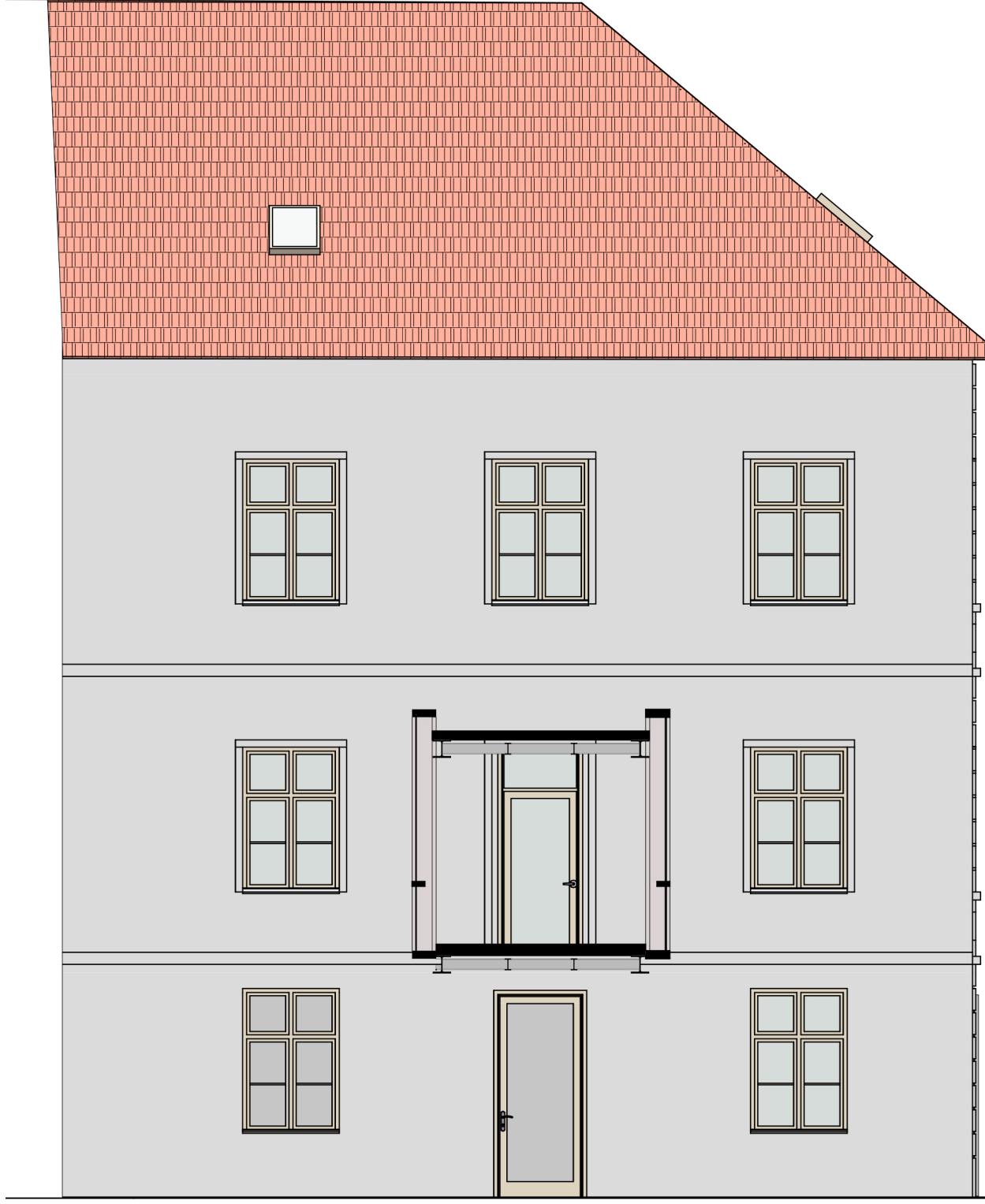
ZÁPADNÍ POHLED A PODÉLNÝ REZ / WESTERN VIEW AND LONGITUDINAL SECTION
