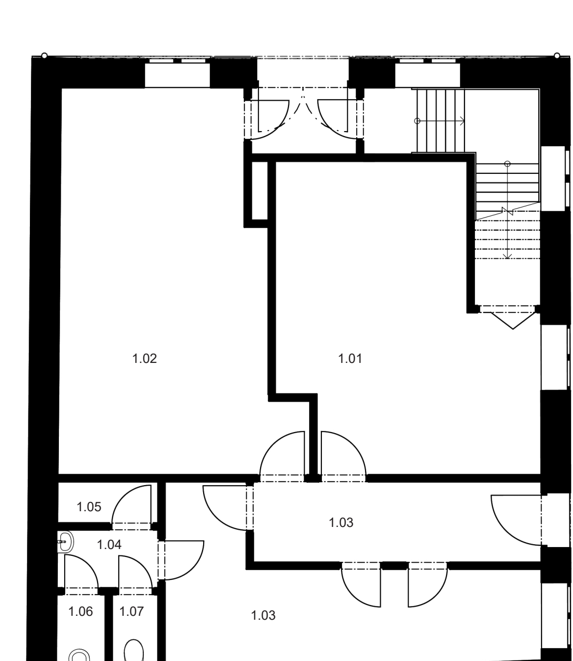
SOUČASNÁ SITUACE OBJEKTU A PŮDORYS 1. NP PŘED ZÁSAHEM / CURRENT SITUATION + FLOOR PLAN PRIOR TO THE INTERVENTION
