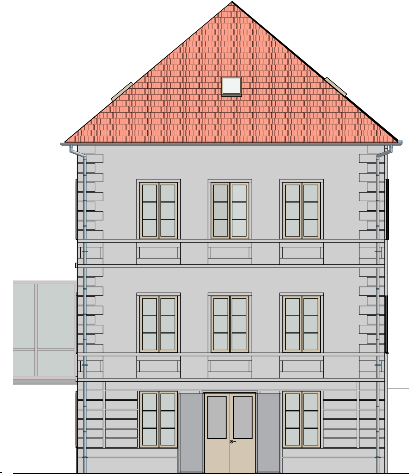
SEVERNÍ POHLED A PŘÍČNÝ REZ / NORTH VIEW AND CROSS SECTION
