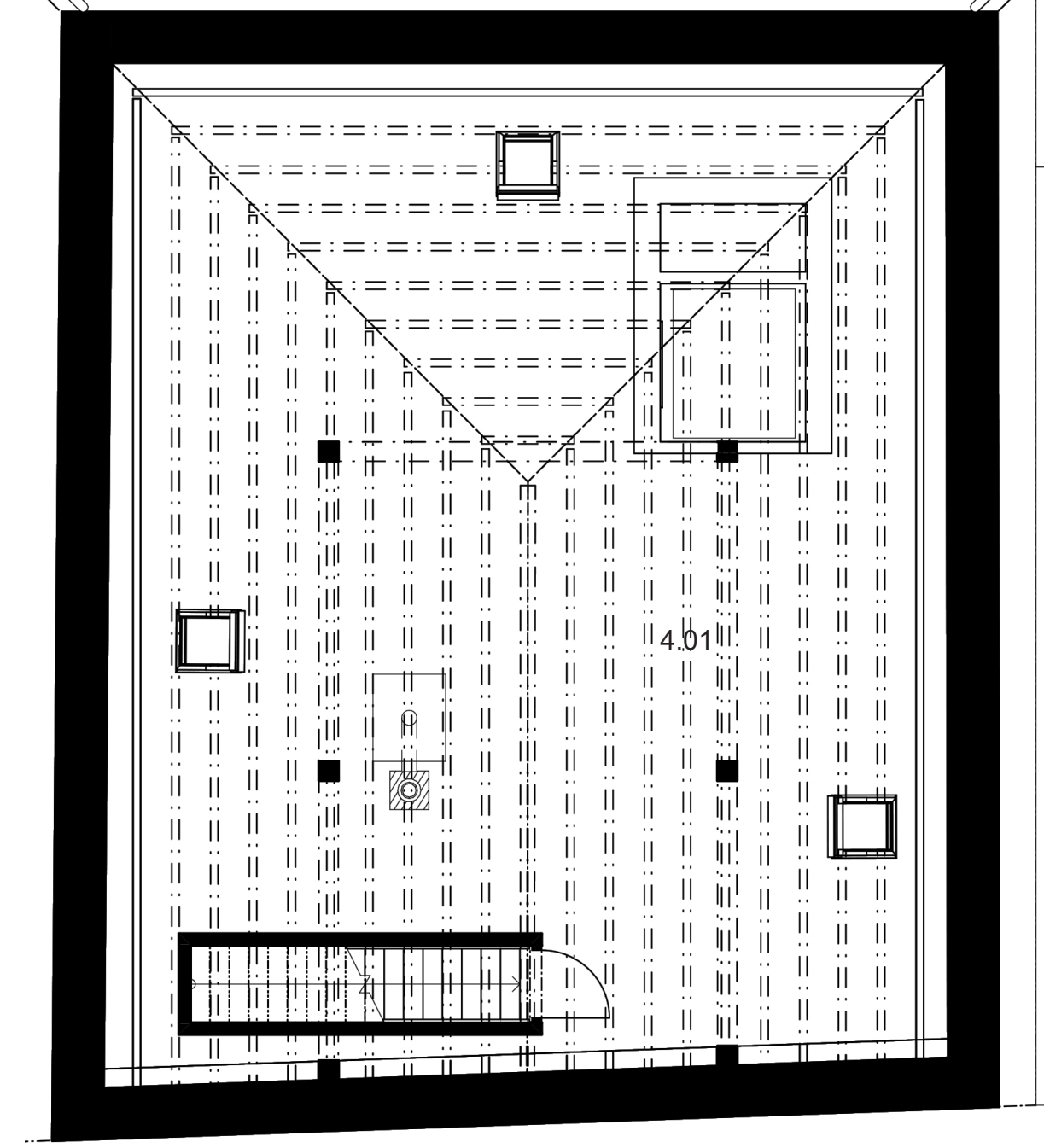
PŮDORYS PODKROVÍ / ATTIC FLOOR PLAN
